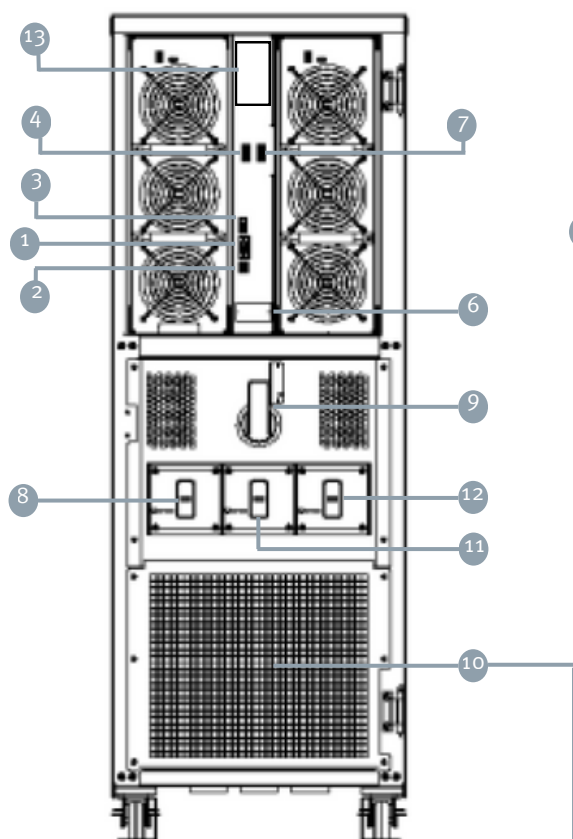
80kVA, 100kVA & 120kVA Models
